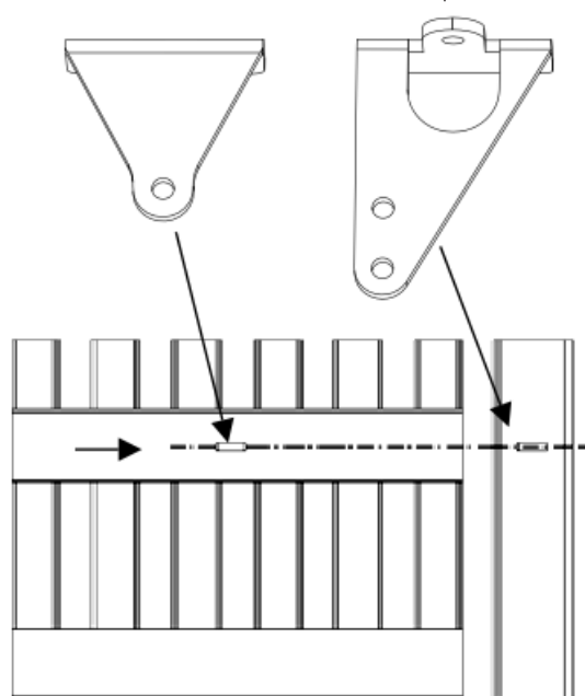
Piastra anteriore Piastra posteriore
